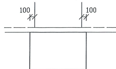
ZÁKLAD POD DVEŘNÍM OTVOREM - POHLED FUNDAMENT UNTER TÜRFÖFFNUNG - ANSICHT
